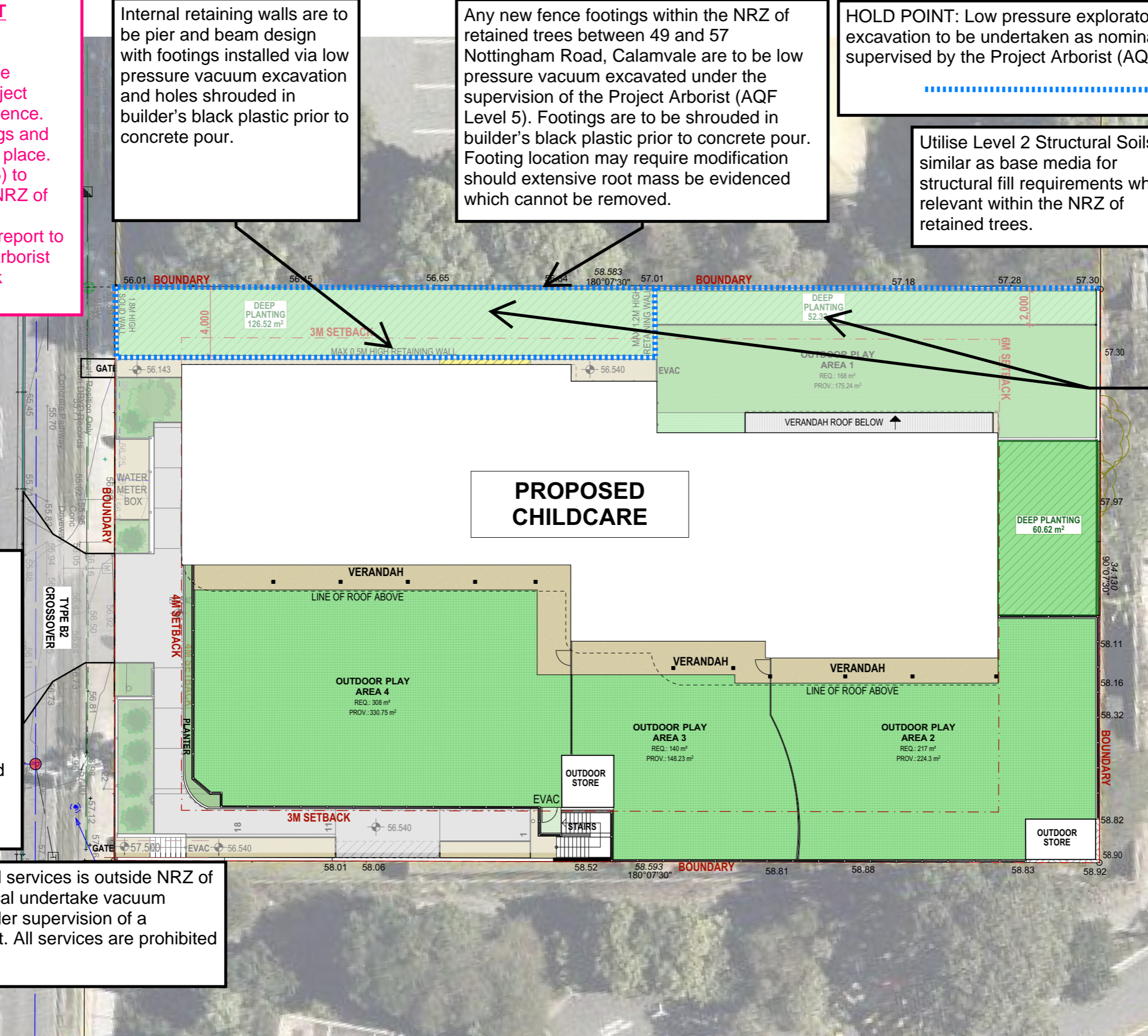
1 SITE PLAN 1:250
