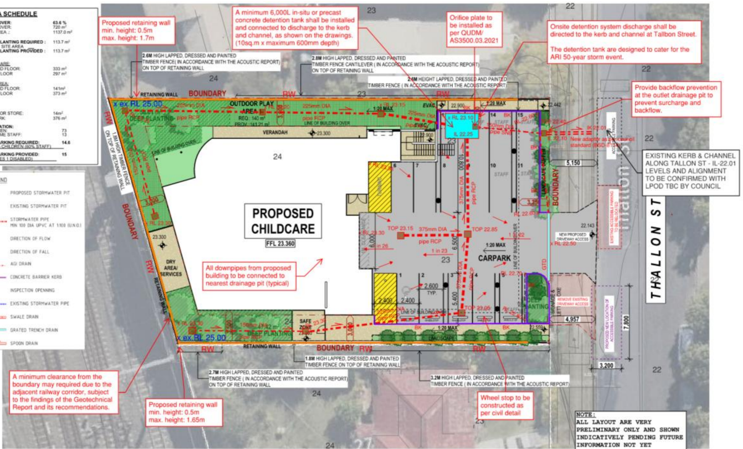
1 SITE PLAN 1:200
